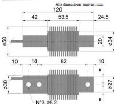
Montagetillbehör KFXC
