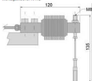
Montagetillbehör KFXC
