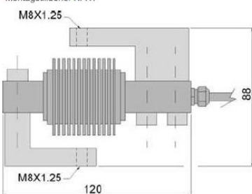
Montagetillbehör KFXT
